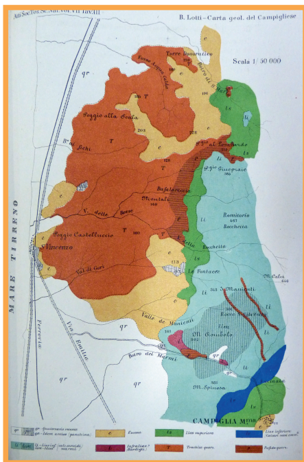
Carta geologica monti di Campiglia (Bernardino Lotti)
